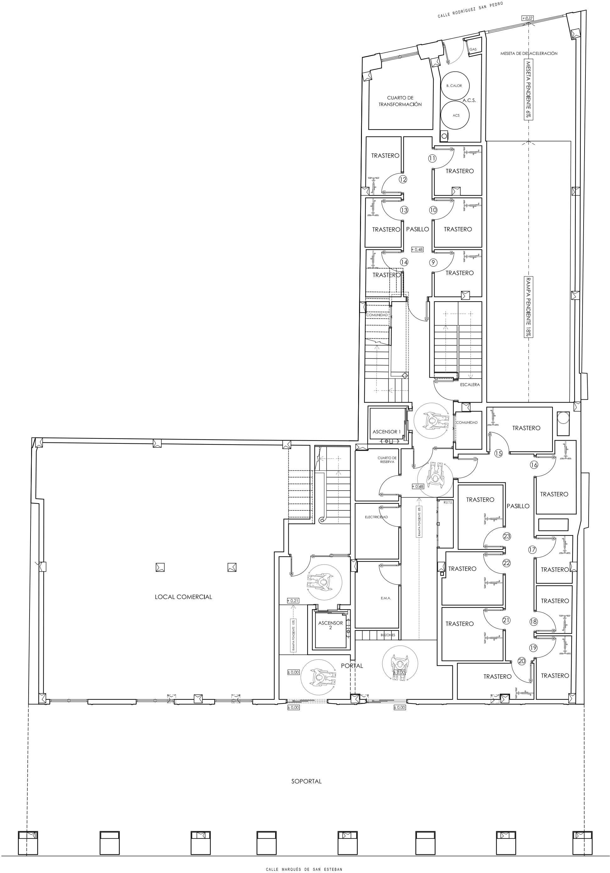
PLANTA BAJA
